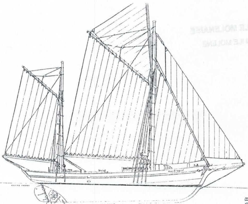
Le « Martroger III » : 17,04 m de long pour 5 m de large et un tirant d'eau de 2,10 m.
